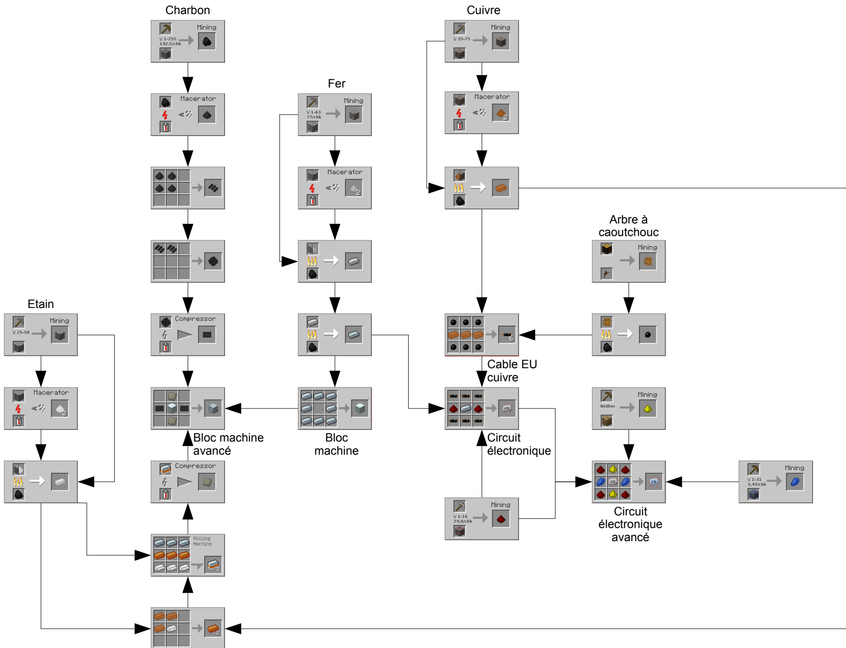
Composants communs de machines (EU)
